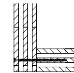
Rechtwinkliger Stumpfstoß
