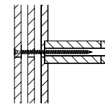
Einglassener Stoß, Vollgewindeschrauben senkrecht von außen
