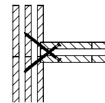
Einglassener Stoß, Vollgewindeschrauben schräg von innen
