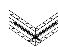
Schräger Stumpfstoß
