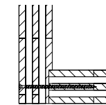
Einglassener Wandstoß
