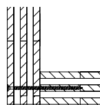
Rechtwinkliger Stumpfstoß
