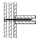
Einglassener Stoß, Vollgewindeschrauben senkrecht von außen
