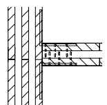
Stumpfstoß, einglassene Winkel und Kammnägel / Schrauben
