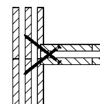
Einglassener Stoß, Vollgewindeschrauben schräg von innen
