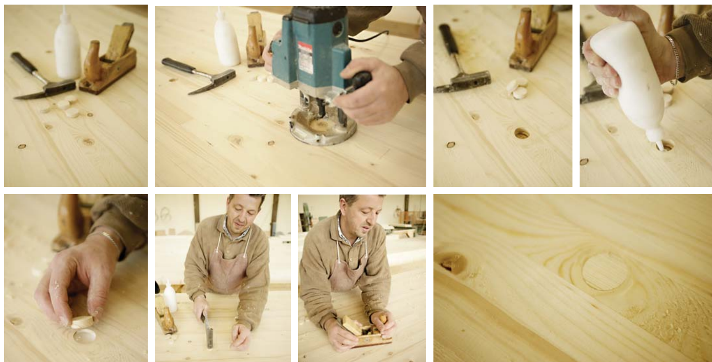
Bild 4a-h Ausbessern von Ästen durch Astlochstopfen
